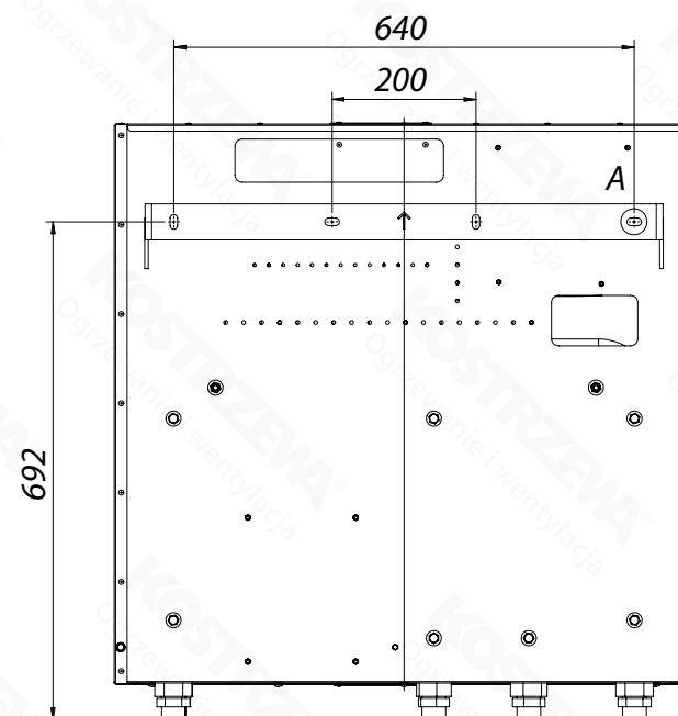
ROZSTAW OTWORÓW MONTAŻOWYCH
