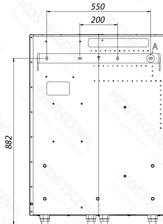
ROZSTAW OTWORÓW MONTAŻOWYCH
